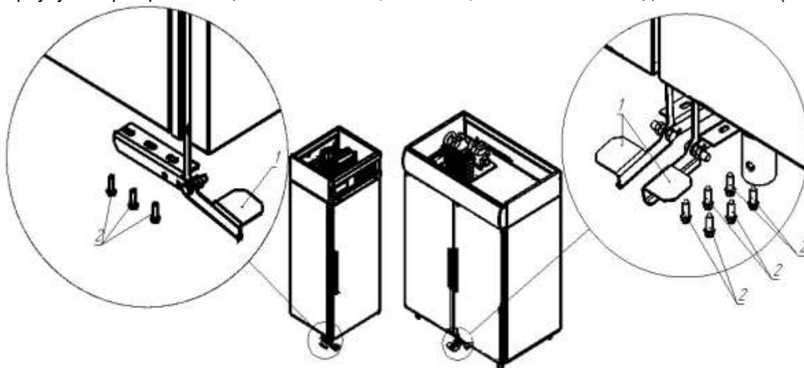
Рис.2 Установка педалей
